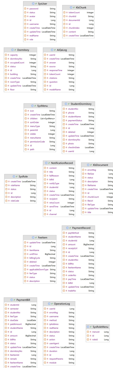
图 3-1 实体类图
