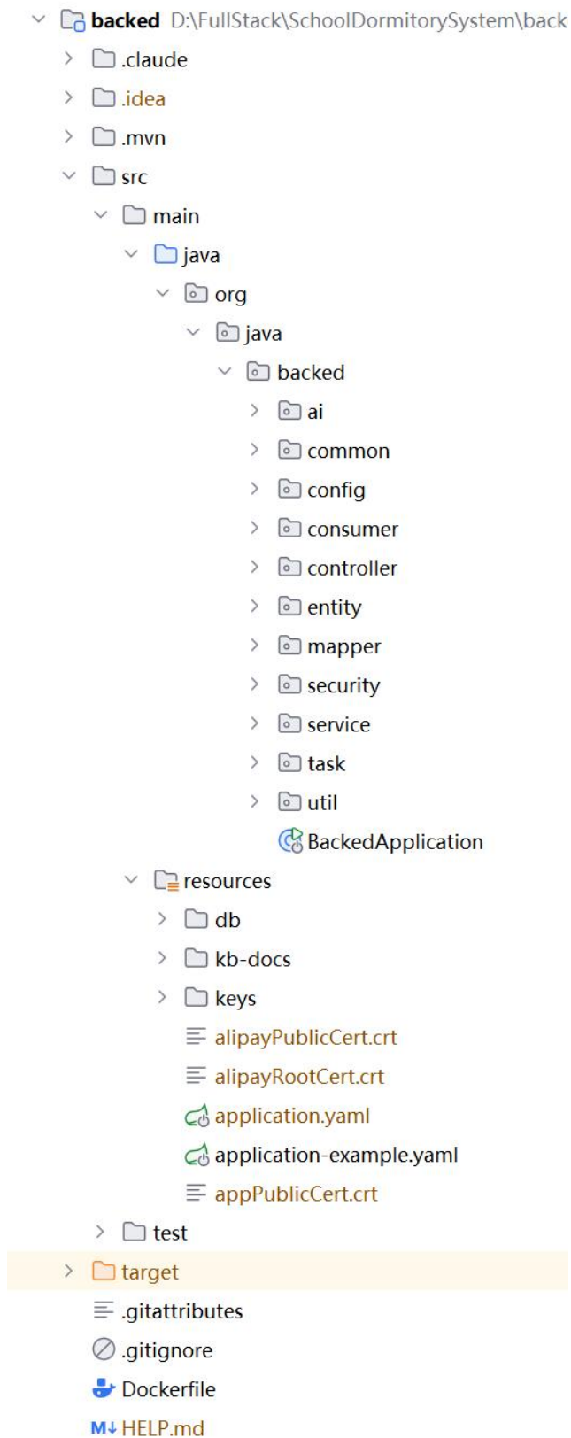
图 2-1 SpringBoot 架构图
